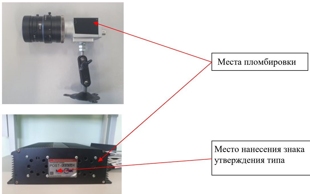
Рисунок 2 – Места нанесения знака утверждения типа и пломбировки от несанкционированного доступа комплексов
